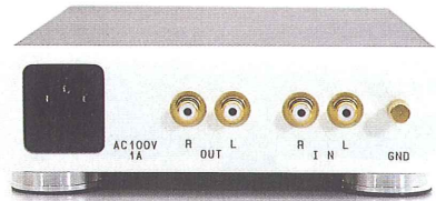
端子はRCAのみ。入力、出力各1系統を装備している
